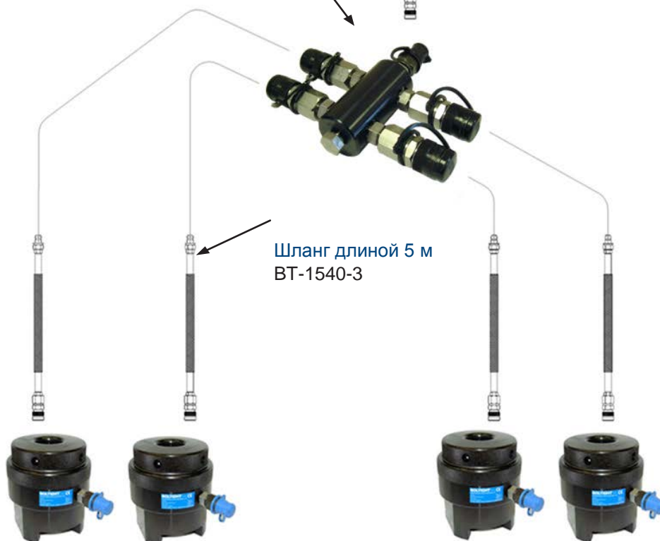
Четырехпортовый распределитель BT-1580
